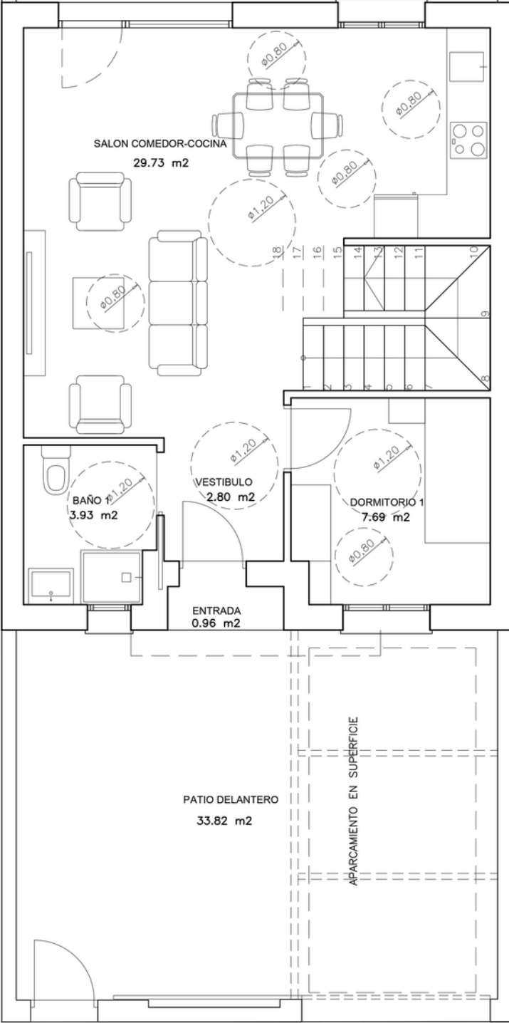
PLANTA BAJA
